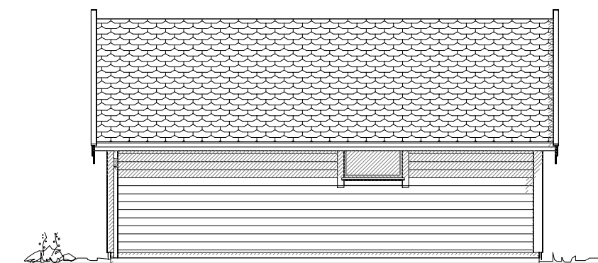
Fasade 2
