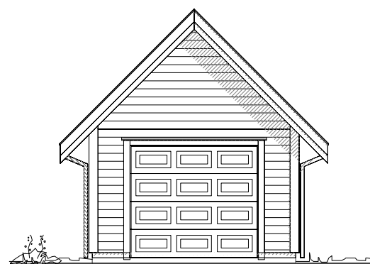
Fasade 1
