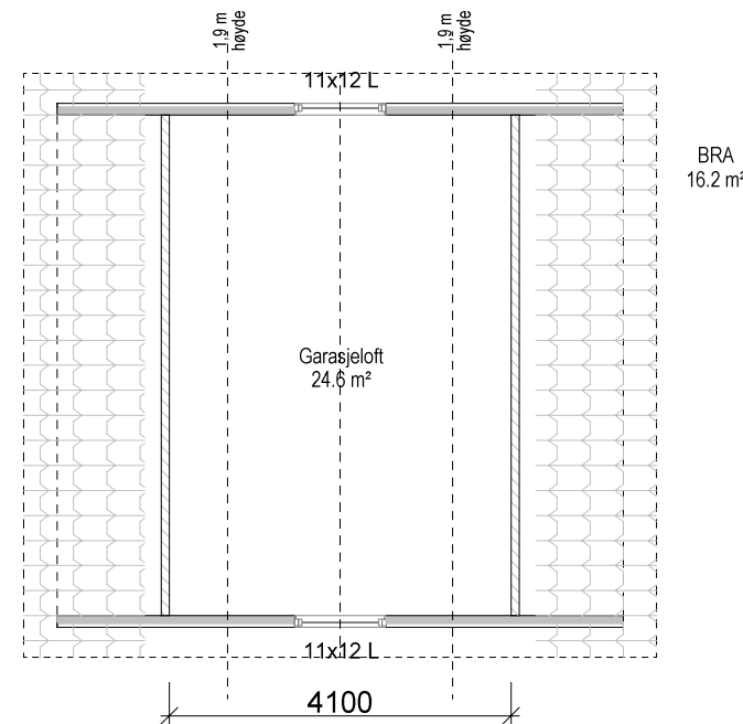
Plan Loft
