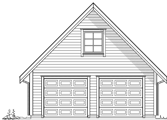
Fasade 1
